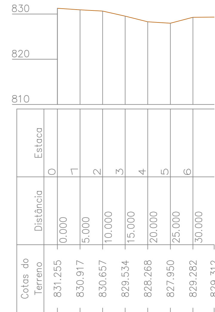
2 PERFIL LONGITUDINAL Escala 1:500
