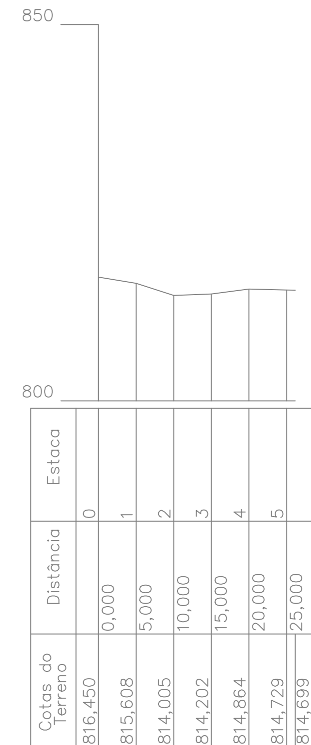
3 PERFIL LONGITUDINAL Escala 1:500
