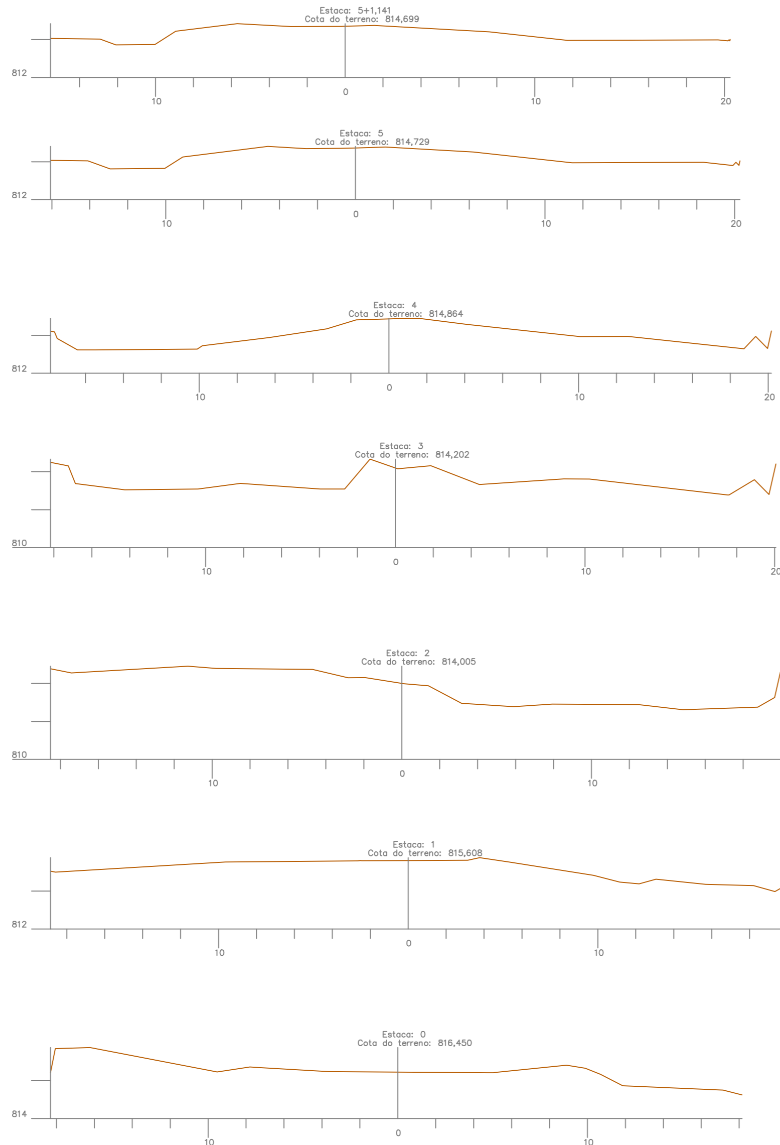
2 SEÇÕES TRANSVERSAIS Escala 1:200
